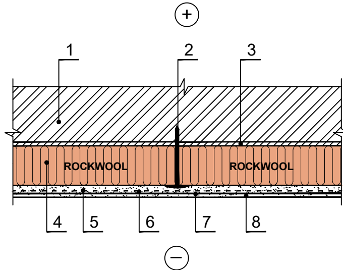
Horizontalus pjūvis
