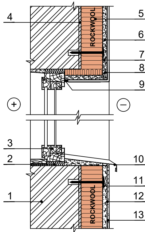
Vertikalus pjūvis
