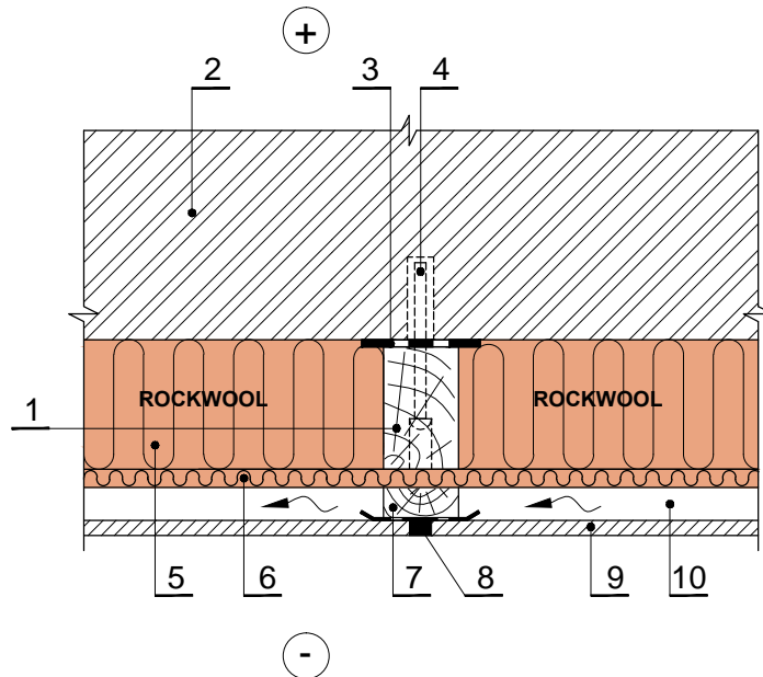
Horizontalus pjūvis
