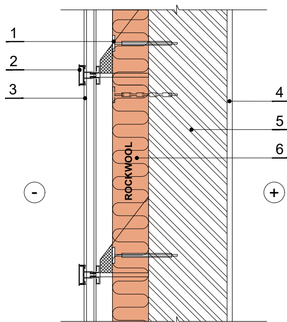
Vertikalus pjūvis
