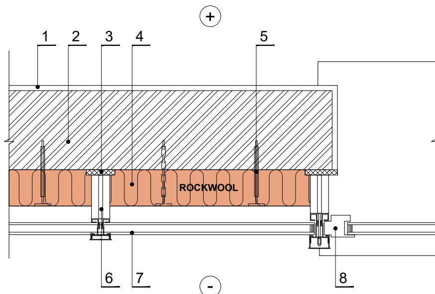
Horizontalus pjūvis
