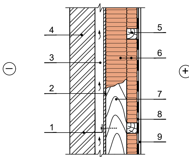
Vertikalus pjūvis
