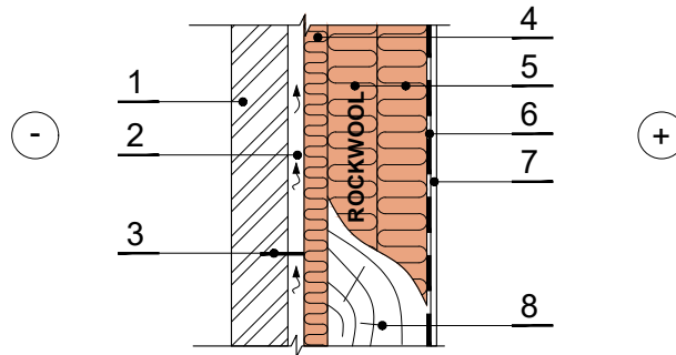
Horizontalus pjūvis
