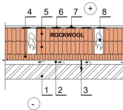
Horizontalus pjūvis
