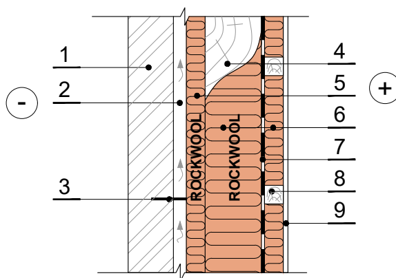
Vertikalus pjūvis
