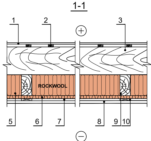
Horizontalus pjūvis
